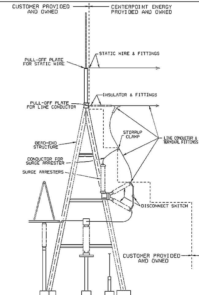
ELEVATION
